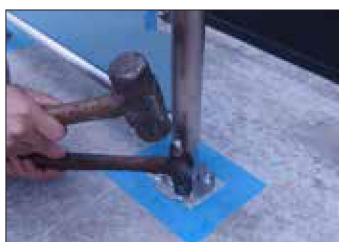
8 本体設置 (アンカーボルト打設)
